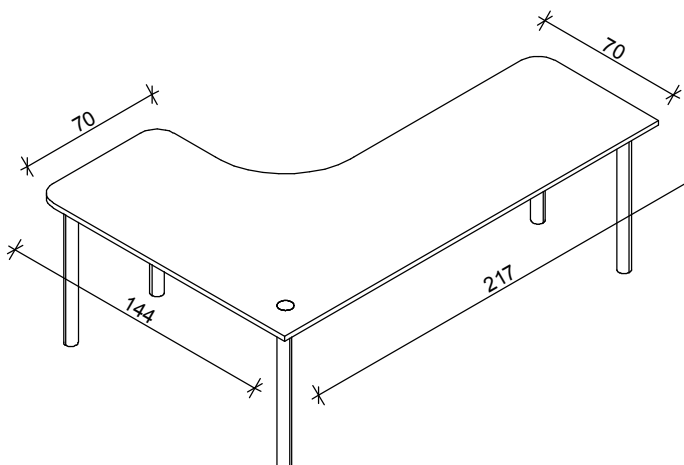
Rys. nr 21 - Biurko narożne, lewe
