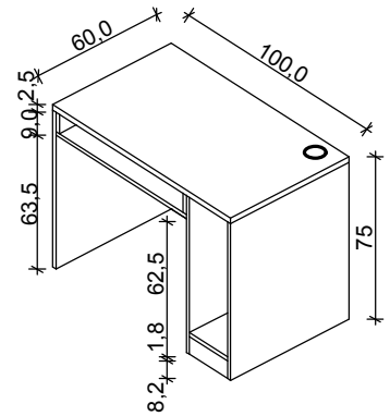
Rys. nr 18 - Biurko proste
