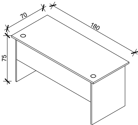
Rys. nr 19 - Biurko proste
