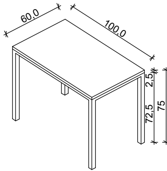
Rys. nr 17 - Biurko proste
