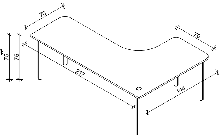
Rys. nr 22 - Biurko narożne, prawe
