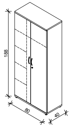
Rys. nr 64 - Szafa gospodarcza
