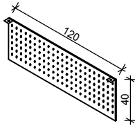
Rys. nr 45 - Osłona przednia
