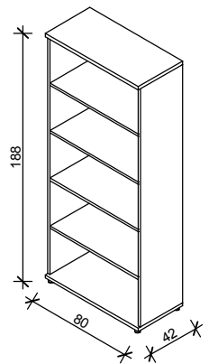
Rys. nr 54 - Regał
