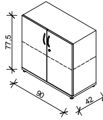
Rys. nr 48 - Szafa biurowa
