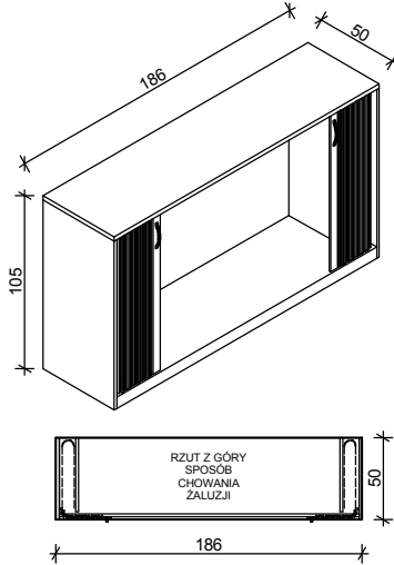
Rys. nr 57 - Regał
