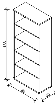
Rys. nr 53 - Regał
