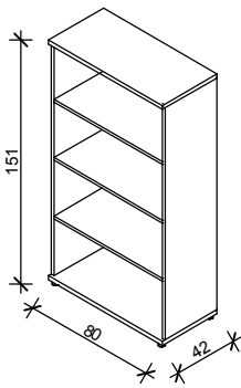
Rys. nr 55 - Regał
