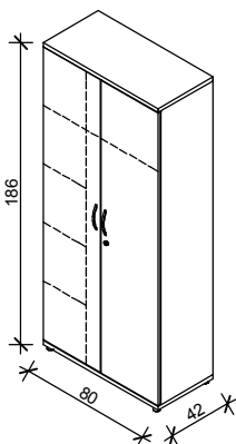
Rys. nr 60 - Szafa ubraniowa
