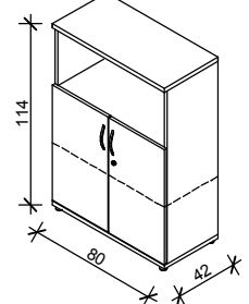
Rys. nr 64 - Szafa gospodarcza
