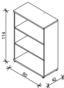
Rys. nr 56 - Regał
