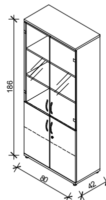
Rys. nr 63 - Szafa biurowa
