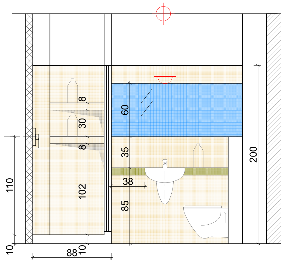
ŁAZIENKA LEWA - WIDOK NA ŚCIANĘ Z UMYWALKĄ
